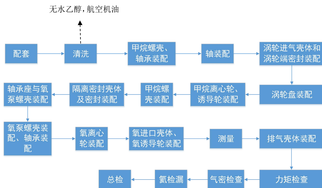
图 5-3 涡轮泵组装及试验流程图
