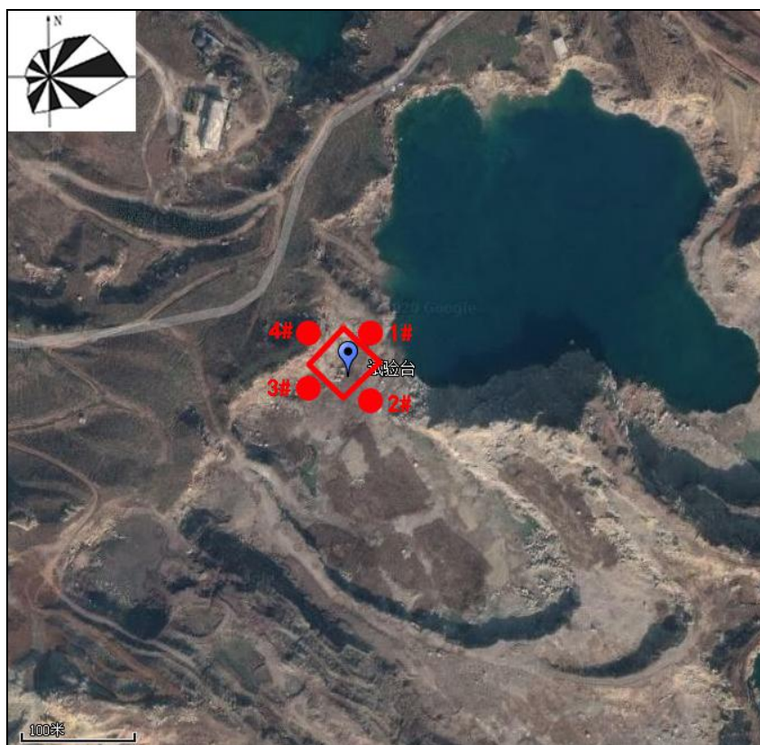
图3-3 试验台噪声监测布点图
