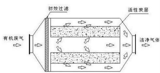
图 7.1-1 活性炭吸附箱
